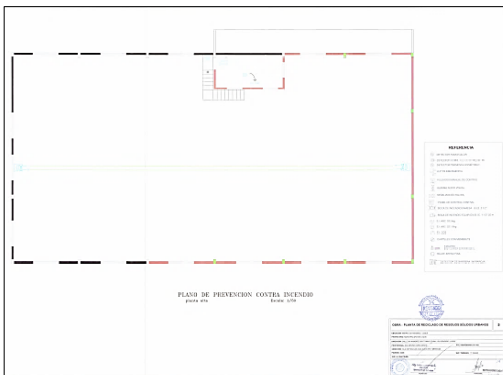
Figura 24. Plano de PCI planta alta aprobado.
