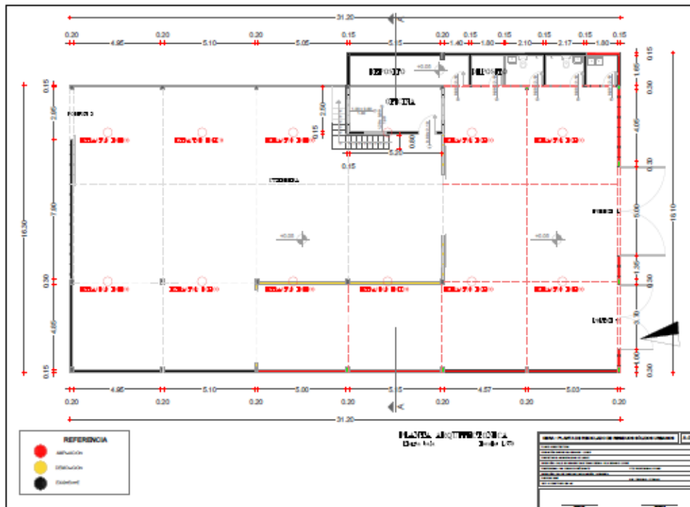
i. Plano A-01 Arquitectura – Planta baja
