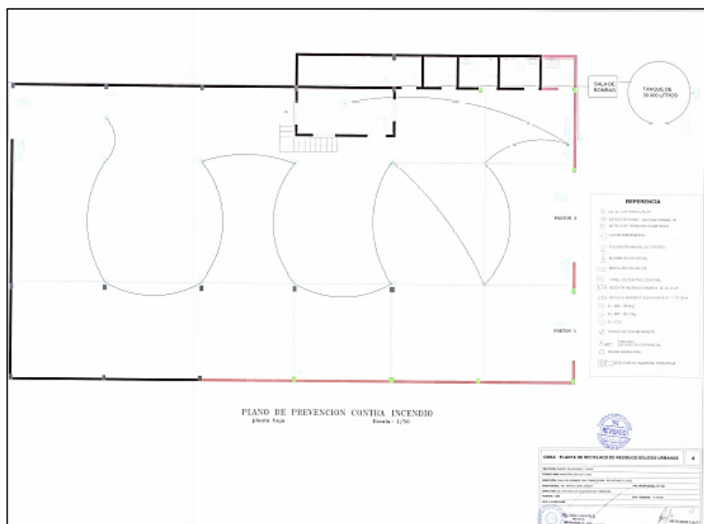
Figura 23. Plano de PCI planta baja aprobado.
