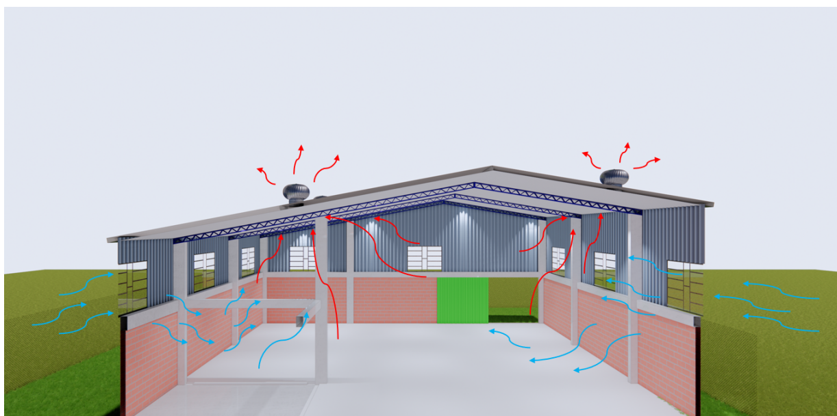
Figura 20. Sentido de ventilación de las áreas.
