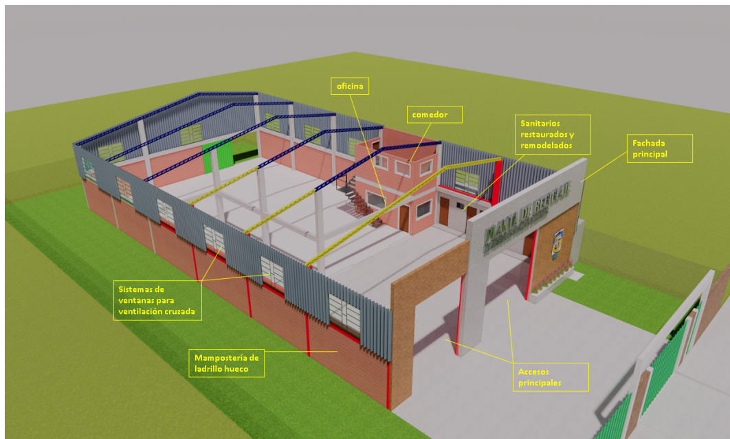
Figura 27. Detalles de paredes y cerramiento
