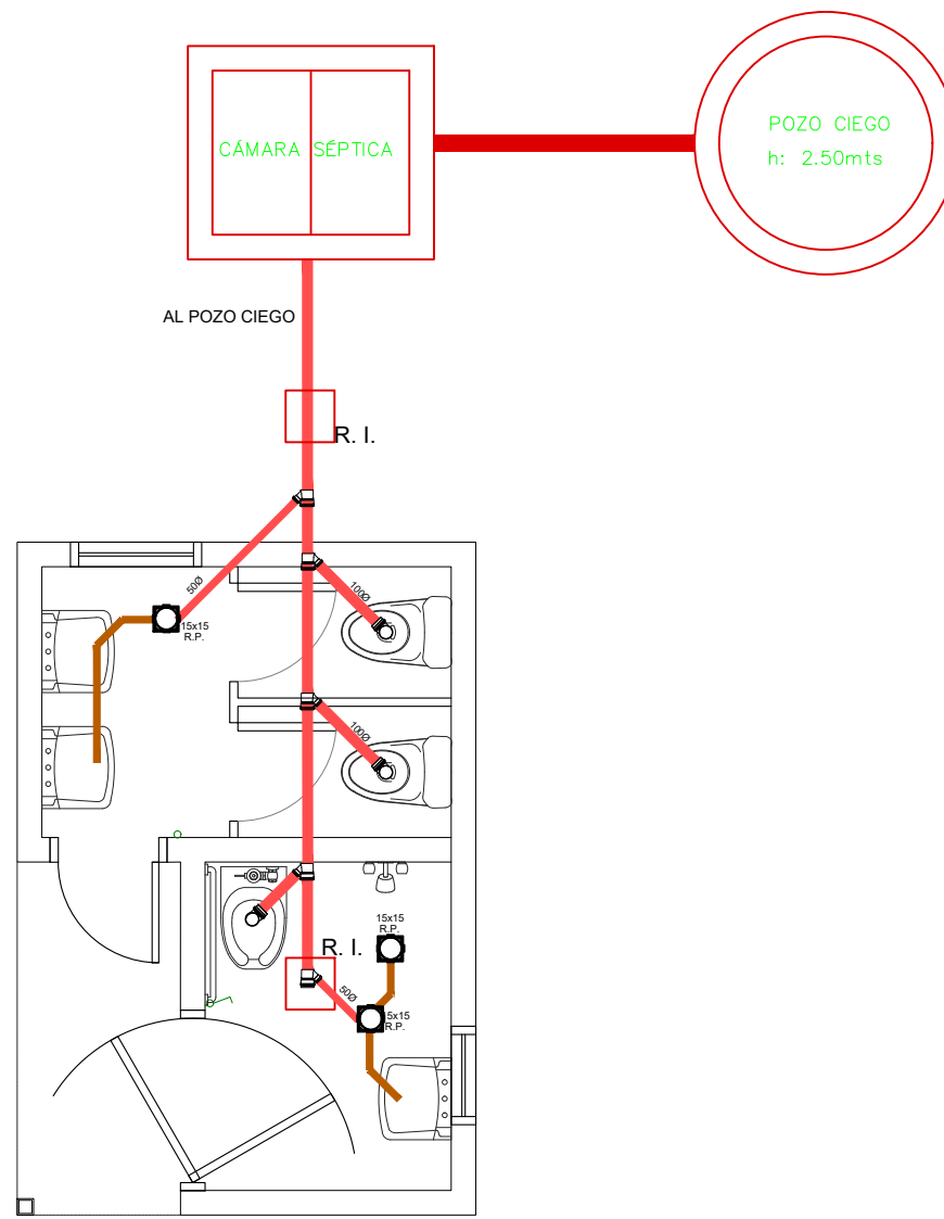
PLANTA DE DESAGUE CLOACAL ESC.: 1/50
