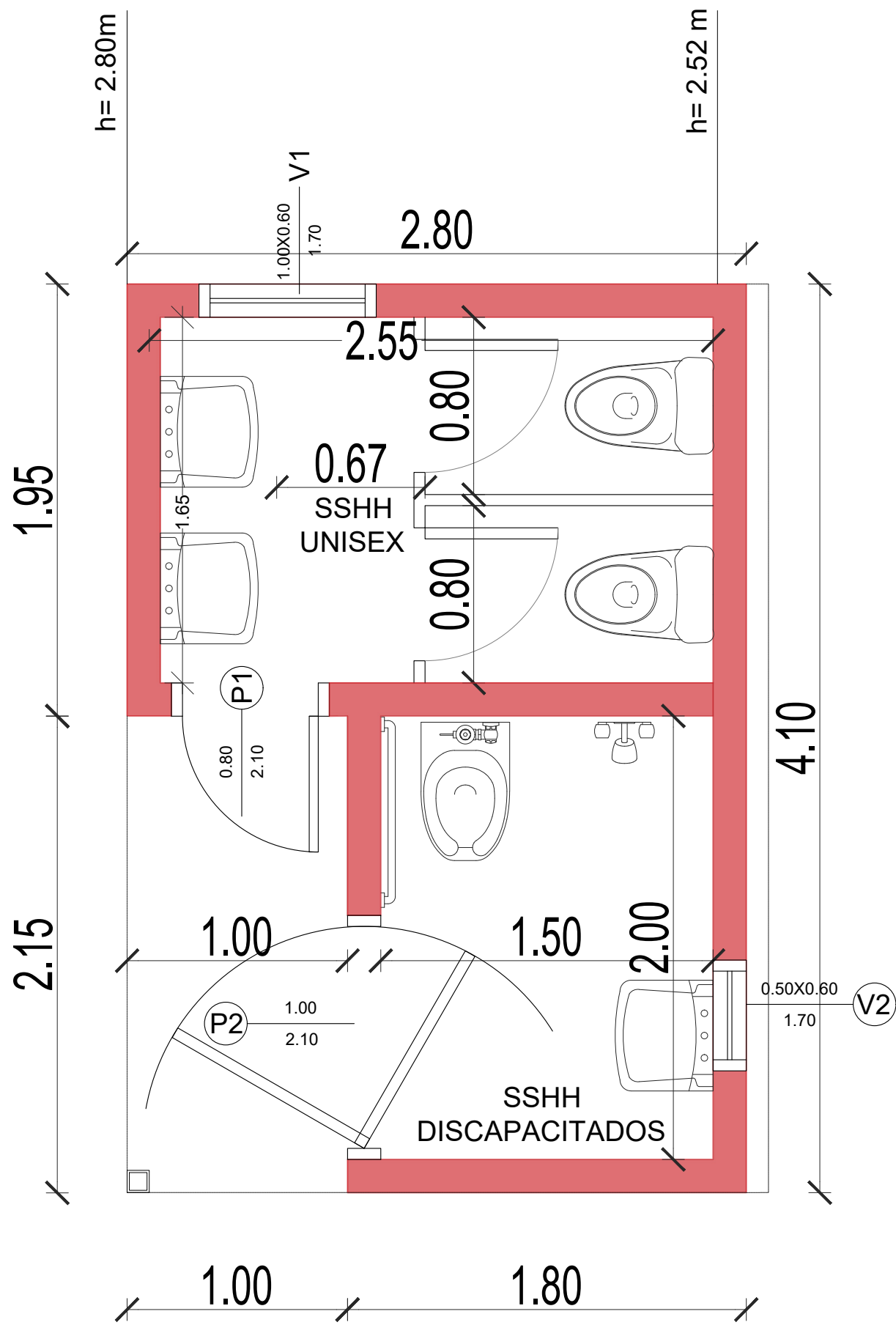
PLANTA ARQUITECTONICA ESC.: 1/25
