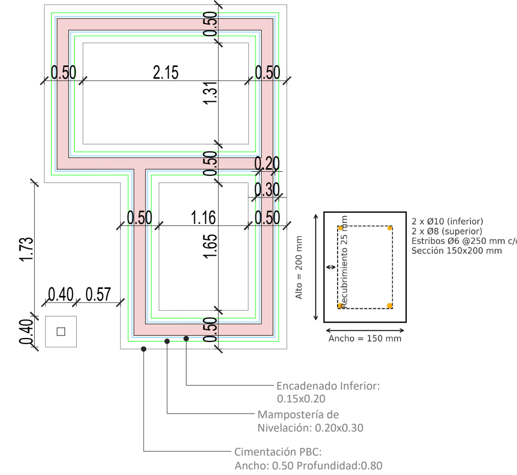
PLANTA DE CIMENTACION ESC.: 1/50
