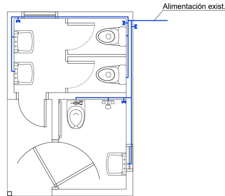
PLANTA DE INST. DE AGUA ESC.: 1/50
